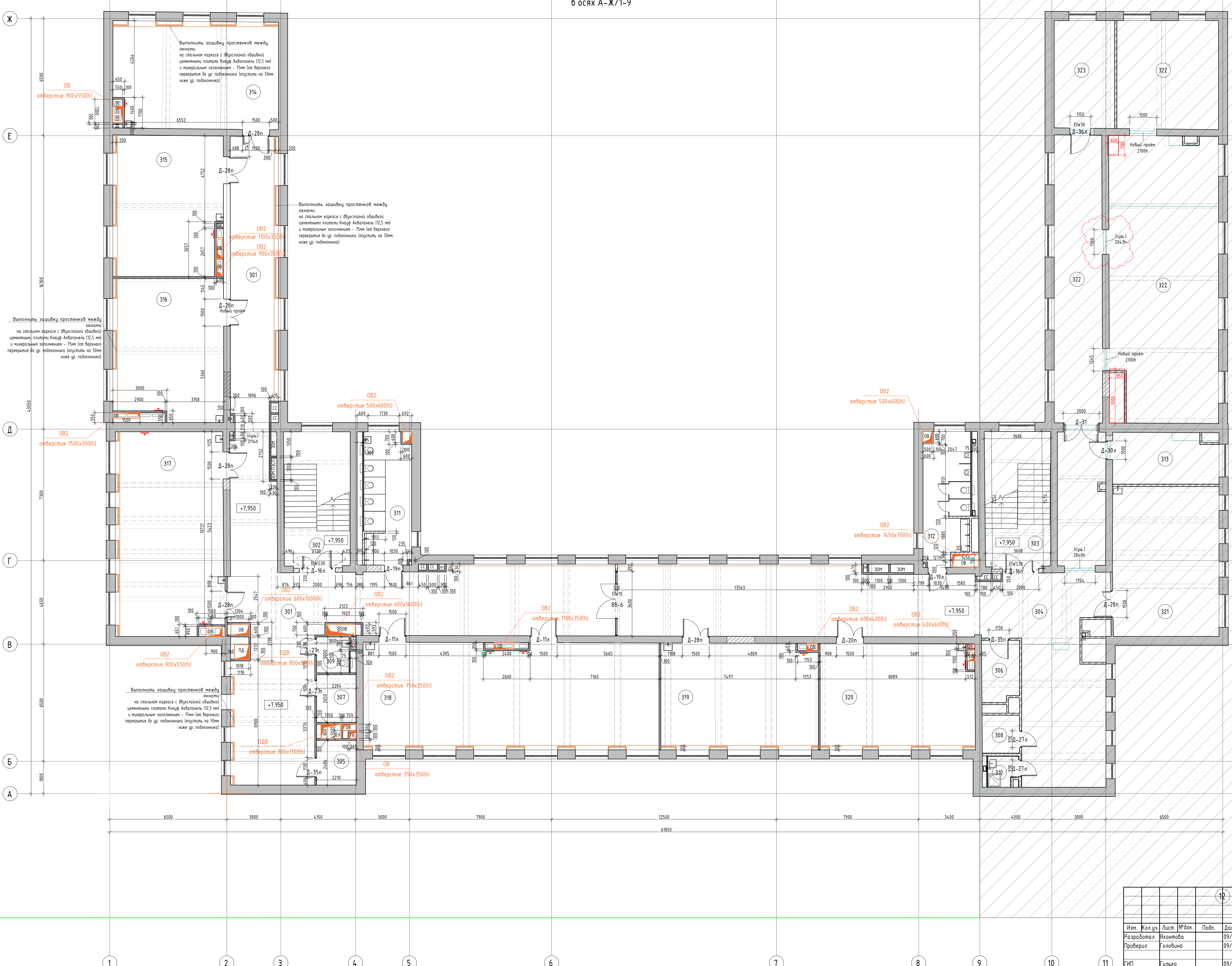
Кладочный план помещений 3-его этажа в осях А-Ж/1-9
